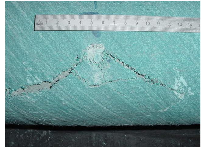
Rohrummantelung nach Prüfung
