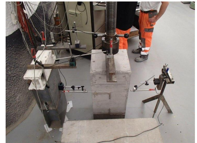
Schubelement
