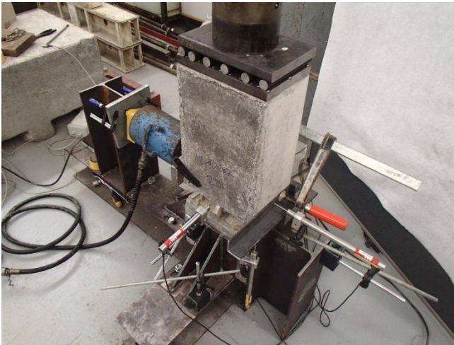
Normalkraftelement mit horizontalem Versatz
