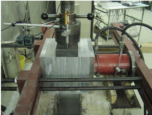
Scherversuch unter Normalkraft an Natursteinplatten
