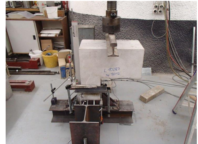
Normalkraftelement mit exzentrischer Krafteinleitung (N-M)
