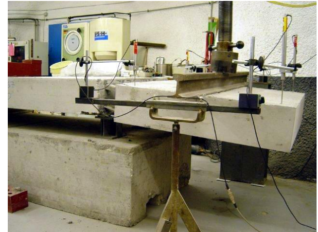
Prüfkörper während dem Versuch
