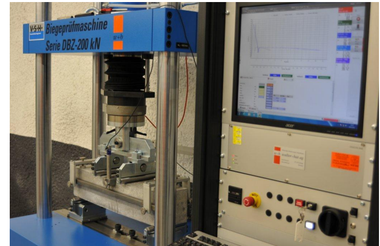
Prüfung Biegezugfestigkeit, deformationsgesteuert
