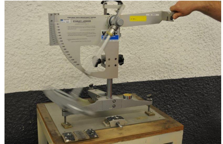
Prüfung Polierwiderstand (PSV)
