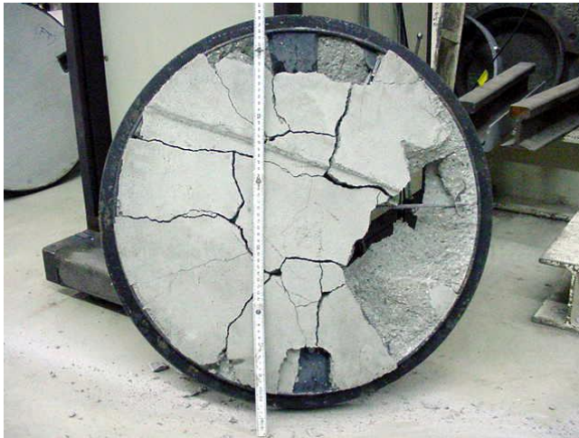
Gussdeckel nach Prüfung
