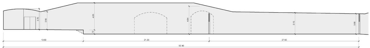
Schnitt A-A, 1:100
